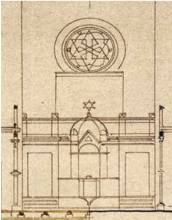
(Abb. 16: erweiterte Synagoge, Ostseite des Inneren mit Toraschrein und Bima)
