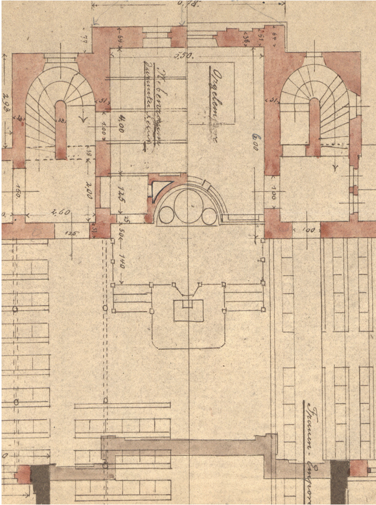
(Abb. 14: erweiterte Synagoge Erdgeschoss)
