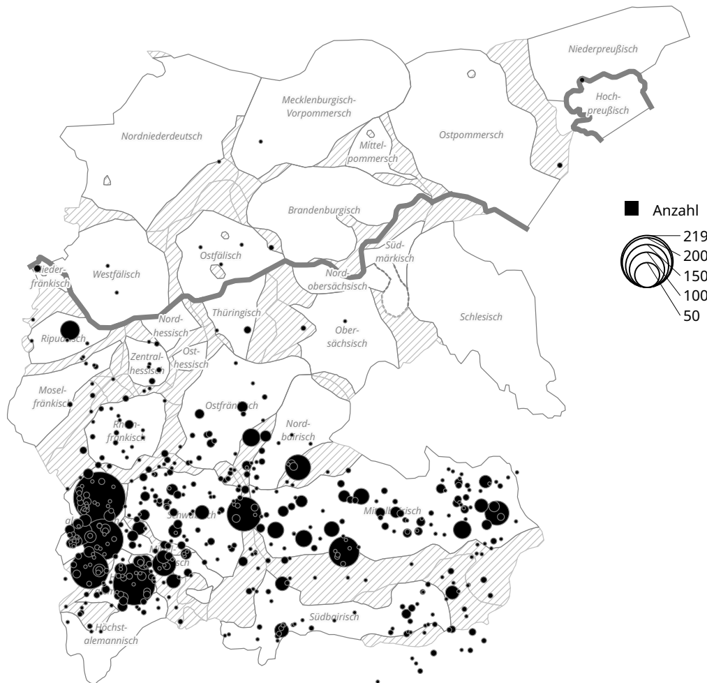
Abbildung 4.1: Urkunden pro eindeutigem CAO-Ausstellungsort (Hintergrund nach Wiesinger 1983: Karte 47.4)
