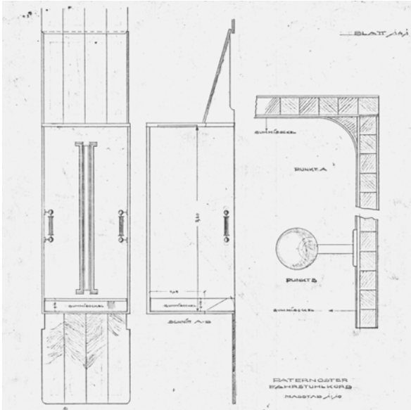
Abb. 4: Nordwollehaus (heute Haus des Reichs), Bremen, Fahrkorbentwurf von Hermann und Eberhard Gildemeister, 1928.
