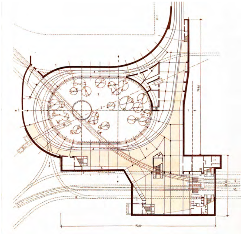
Abb. 5: Kurt Schauss mit Magistratsabteilung 28: Schottenpassage, Grundriss des Untergeschosses, 1961.
