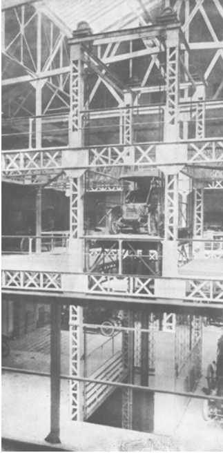
Abb. 4: Garage du Parc Monceau, Paris 1907. Automobilaufzug und hydro-pneumatische Mechanik, Foto 1907.
