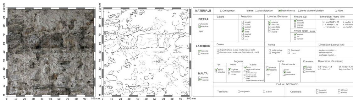
Fig. 35/ Schedatura dell'apparecchiatura muraria interna n. 12.
