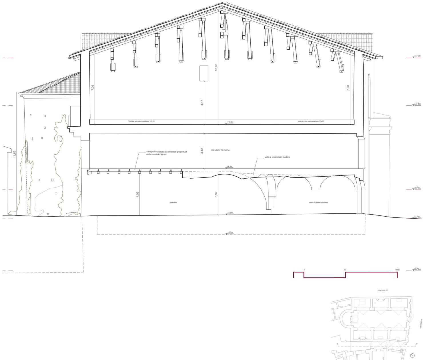
Fig. 35/ Sezione longitudinale GG'.
