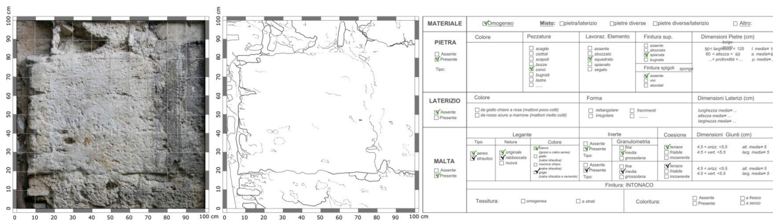
Fig. 32/ Schedatura dell'apparecchiatura muraria interna n. 9.
