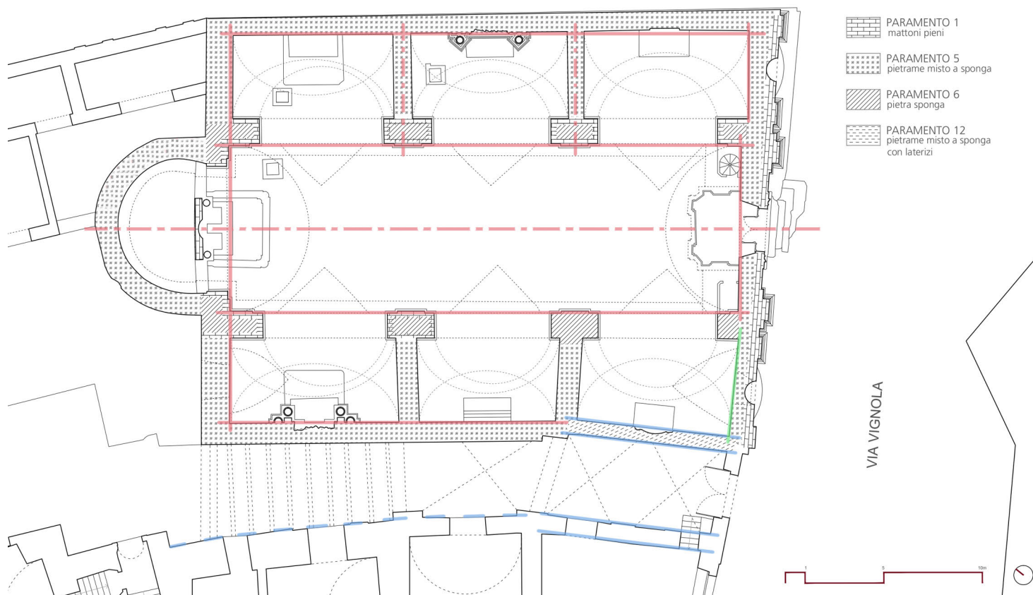
Fig. 7/ Le Apparecchiature murarie e gli allineamenti mostrano la singolarità della prima cappella a sinistra dell'ingresso, frutto di una probabile preesistenza.
