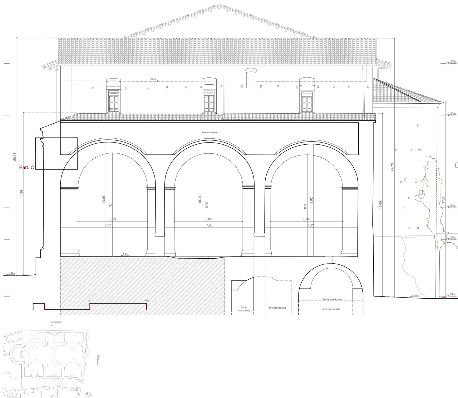
Fig. 32/ Sezione longitudinale DD'. (Particolare cfr. p. 87).
