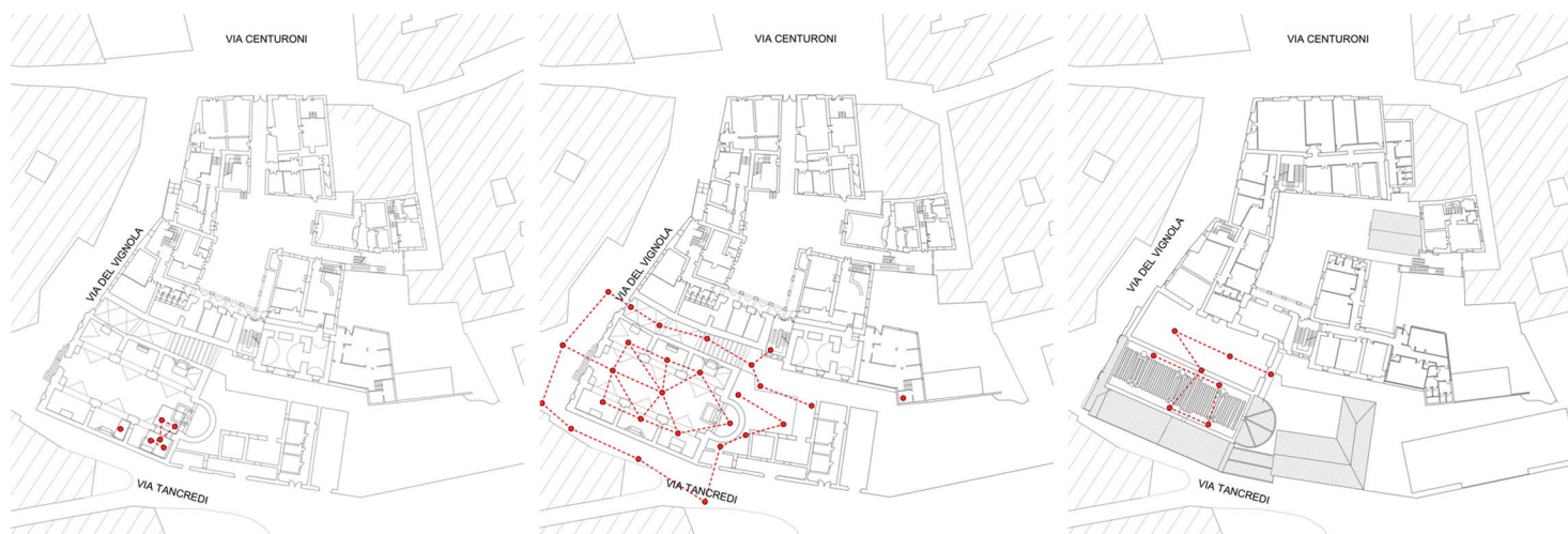
Fig. 6/ Progetto di presa. Sono mostrati tre diversi livelli di acquisizione TLS a quota crescente, a partire dagli ambienti ipogei (a sinistra), superfici esterne e interne della chiesa (al centro), Sala Severi e vano sottotetto (a destra).
