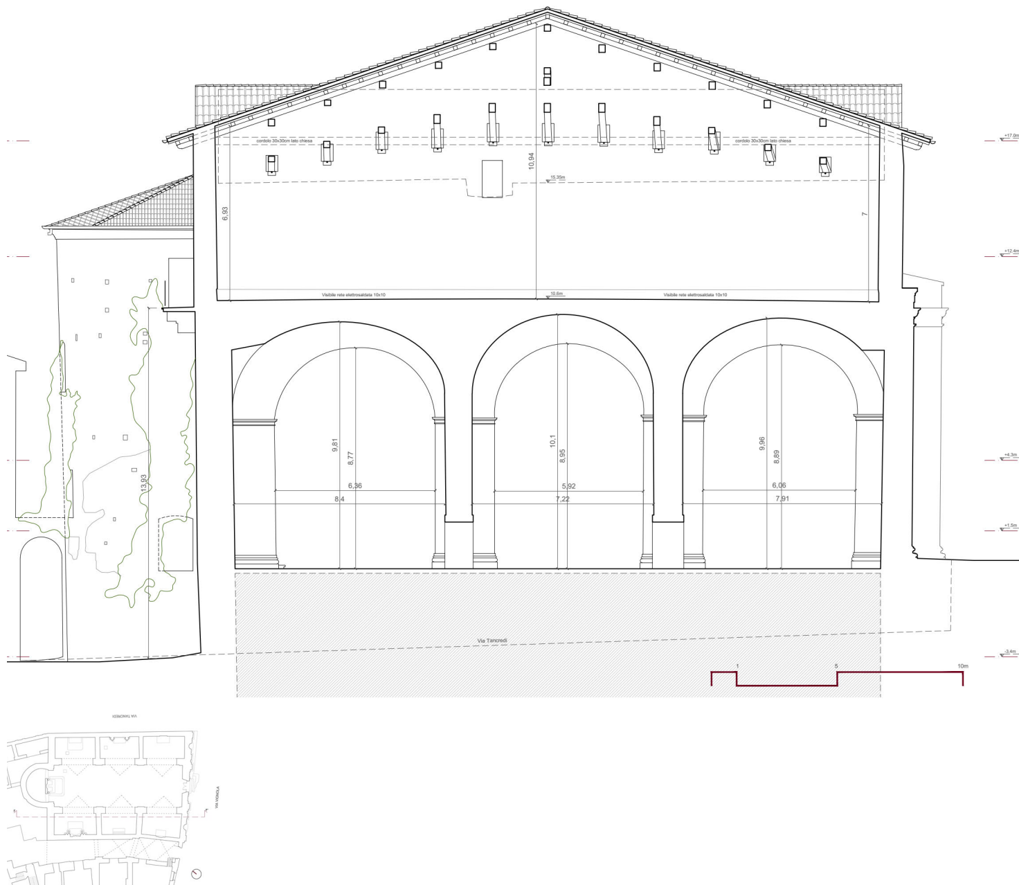
Fig. 34/ Sezione longitudinale FF'.
