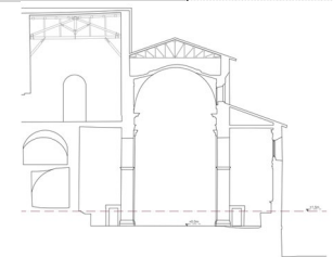
Fig. 21/ Pianta quota +1,50 m.
