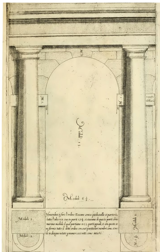
Fig. 8/ Tavola V: porticato con semicolonne addossate senza piedistallo di ordine tuscanico.
