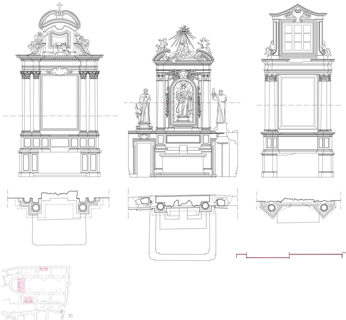
Fig. 48/ Particolari al tratto dell'altare principale e degli altari estradossati.
